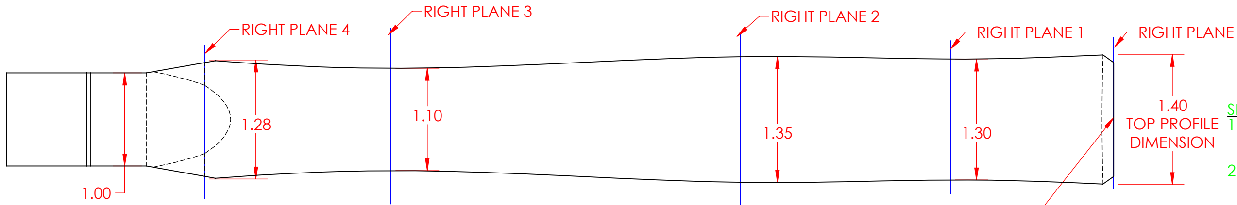
SECTION B-B SCALE 1:1 TOP
